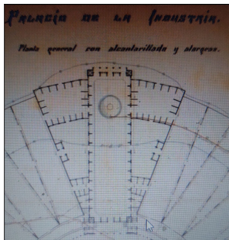
Vista de les naus laterals durant el procés de construcció. Part del plànol del Palau de la Indústria amb les fonamentacions i clavegueres.
